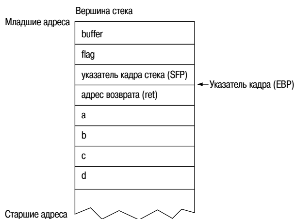
Рис. 2.1. Кадр стека
