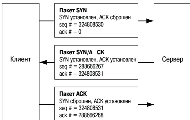
Рис. 4.6. Открытие соединения
