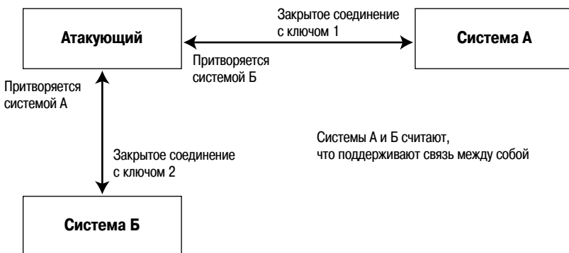
Рис. 7.1. Атака MitM
